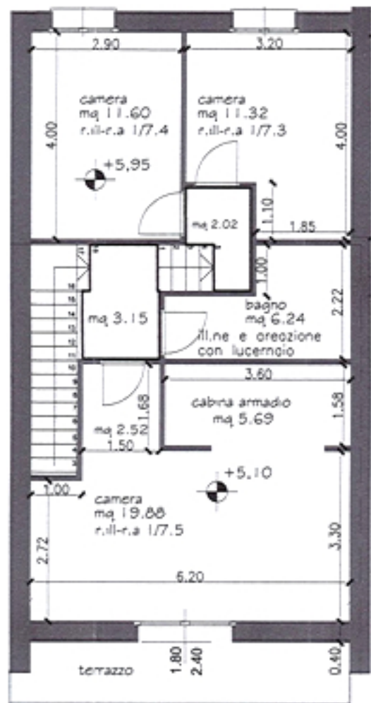
Piano primo
