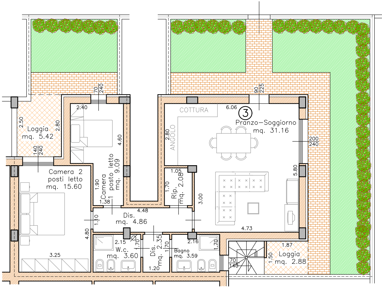
PIANO PRIMO
